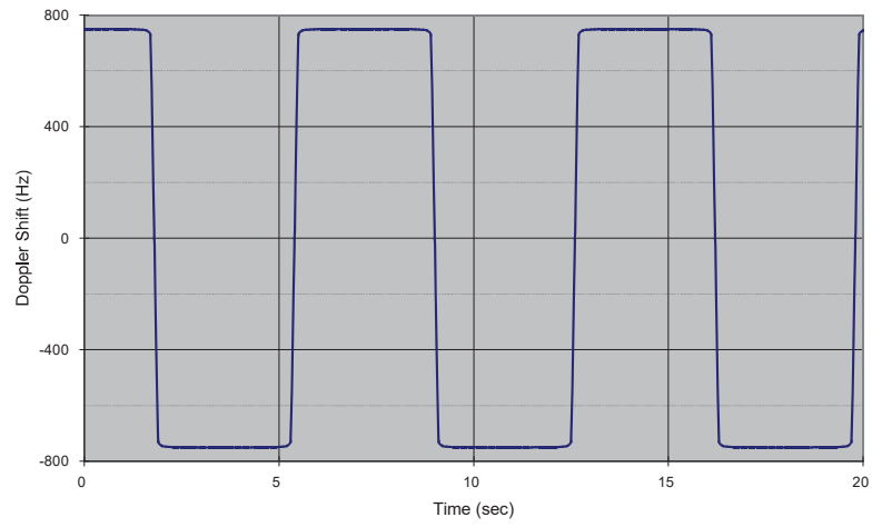
Figure B.3-1: Doppler shift trajectory
