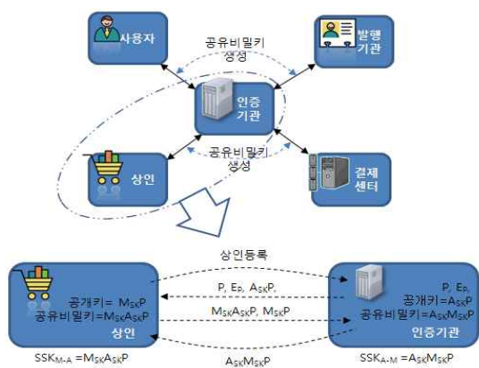
그림 5. 공유비밀키 생성(상인과 인증기관)
