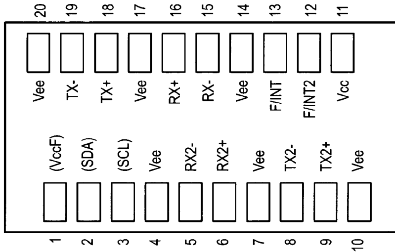
FIG. 15D
