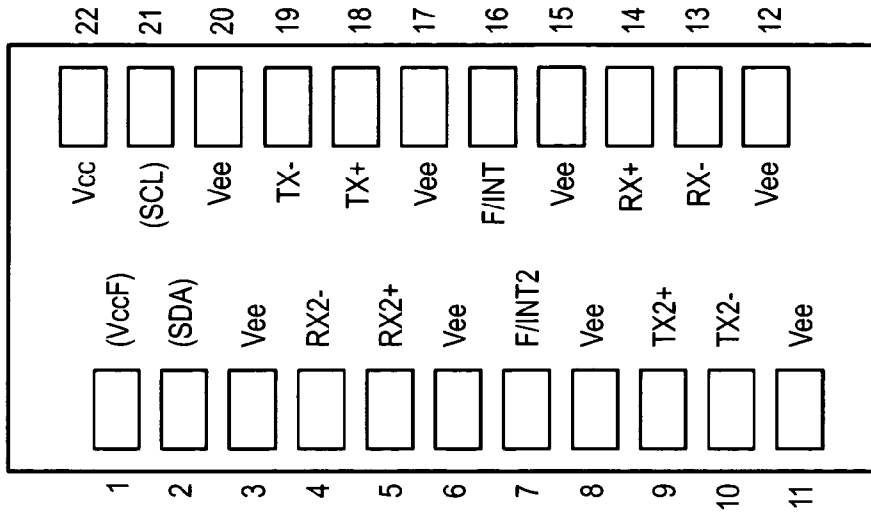
FIG. 15E
