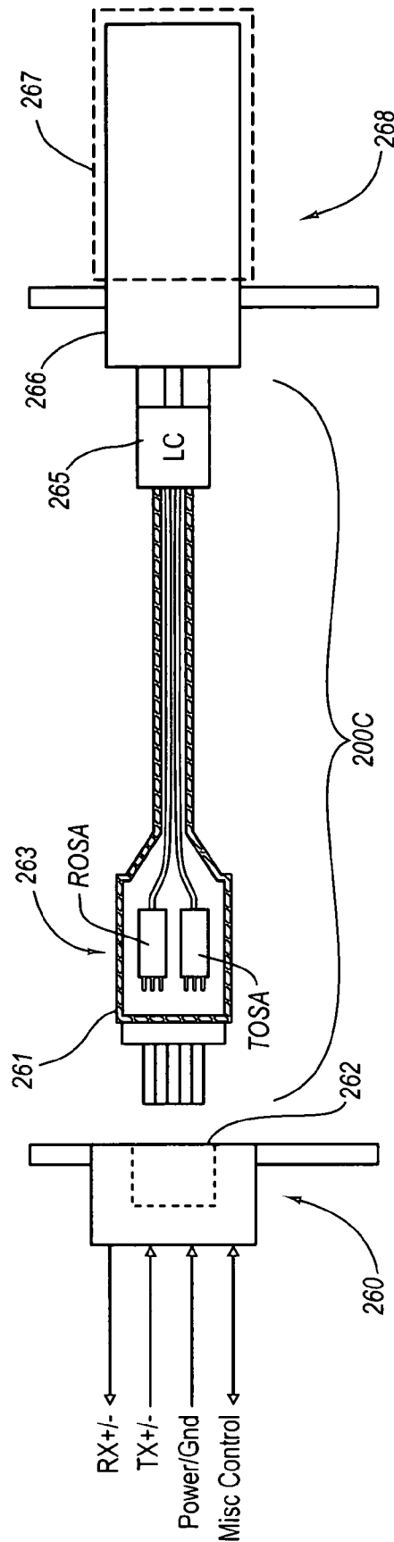
FIG. 2C
