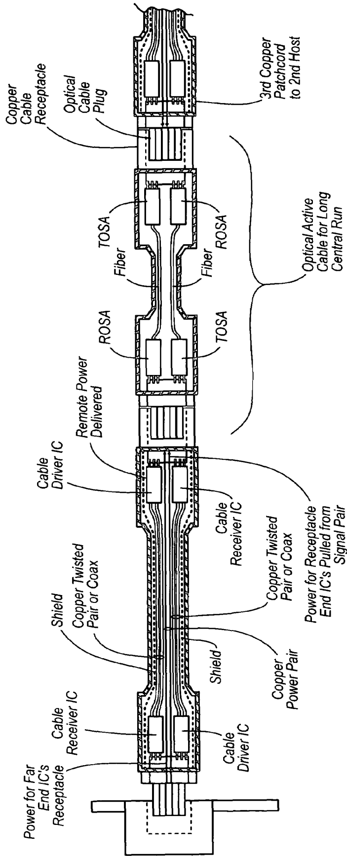
FIG. 13A
