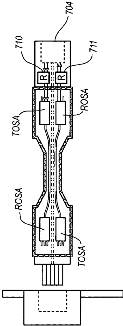
FIG. 7A
