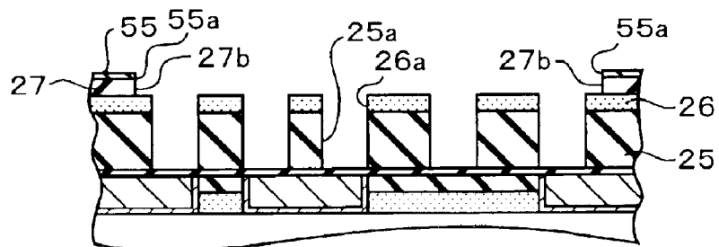
FIG. 12J
