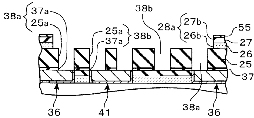
FIG. 12K
