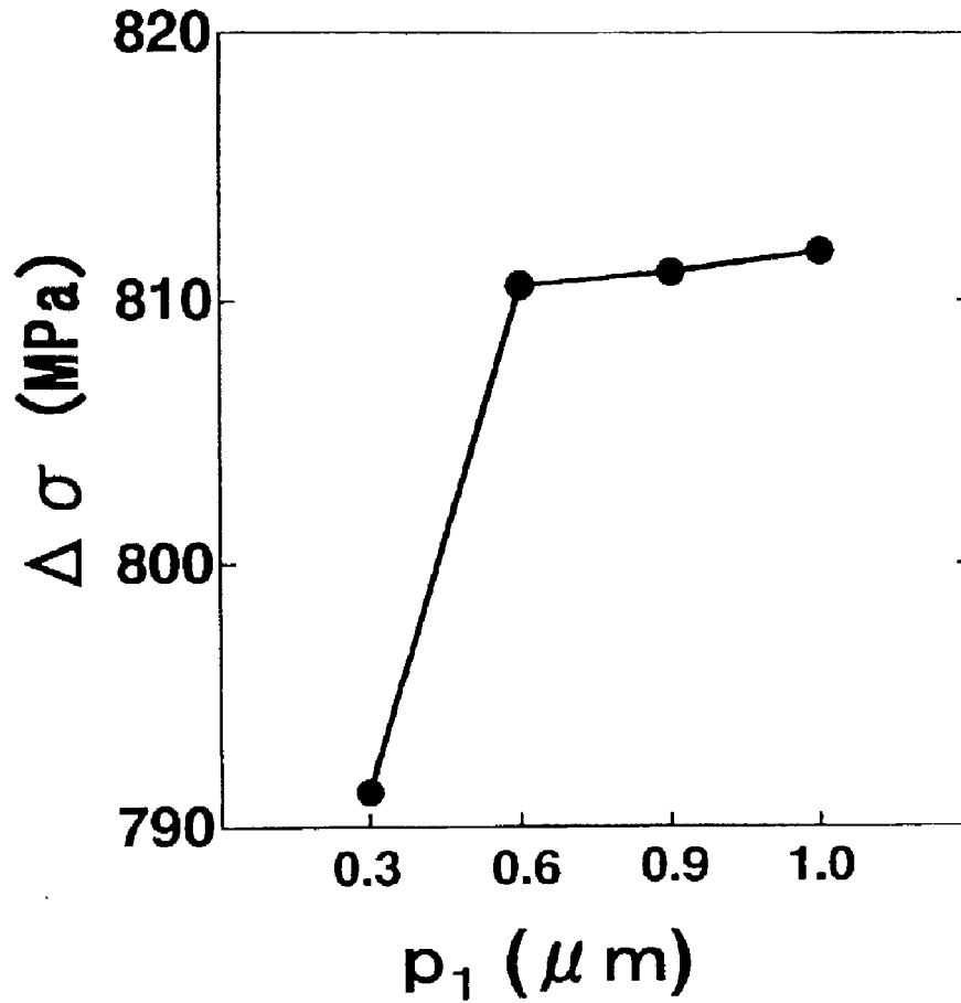
FIG. 15A
