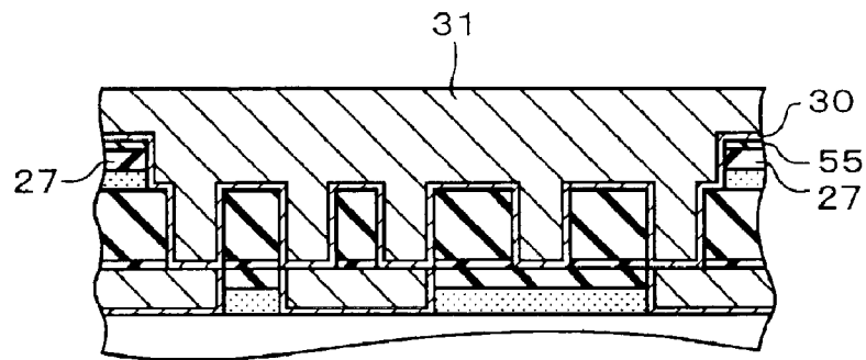
FIG. 12L
