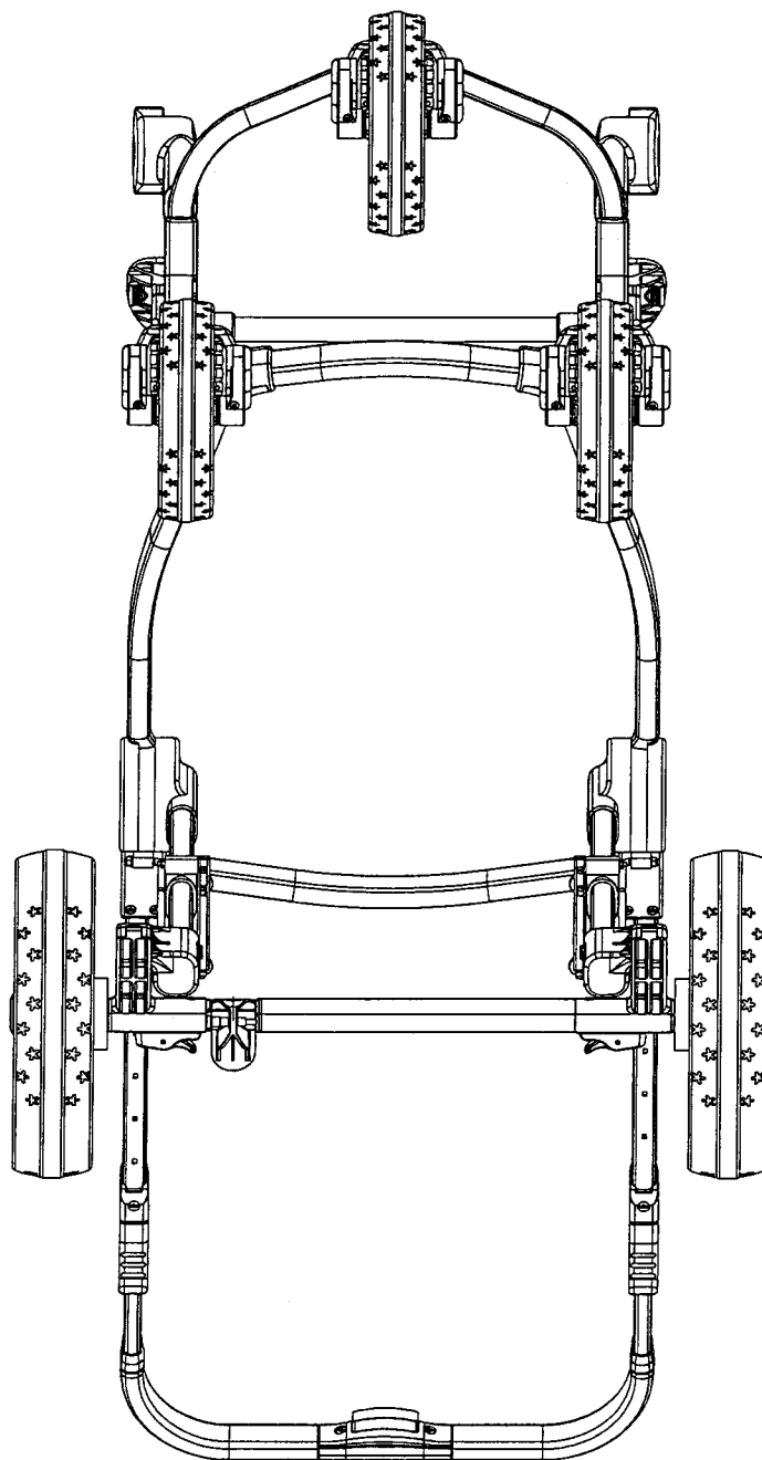
仰視圖
