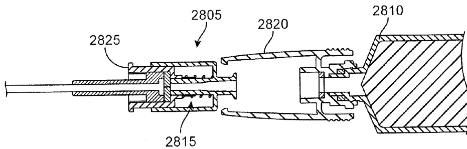
FIG. 27A
