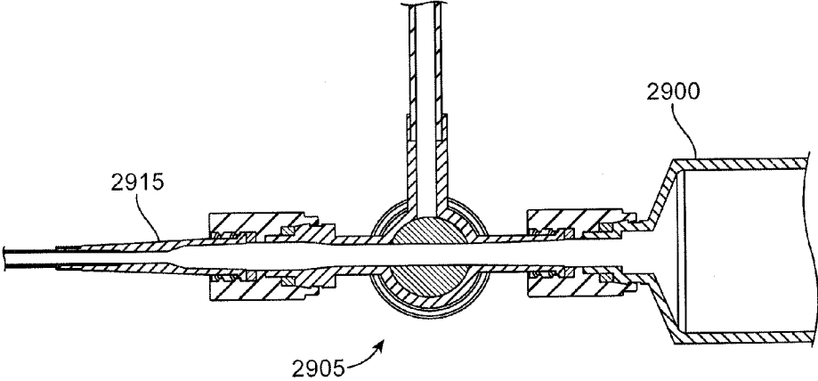
FIG. 29A
