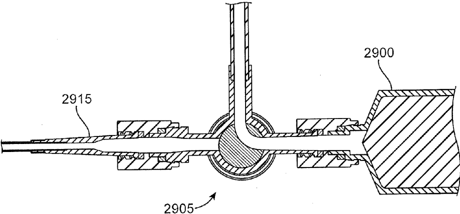
FIG. 29B
