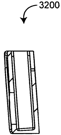
SECTION A-A FIG. 32F
